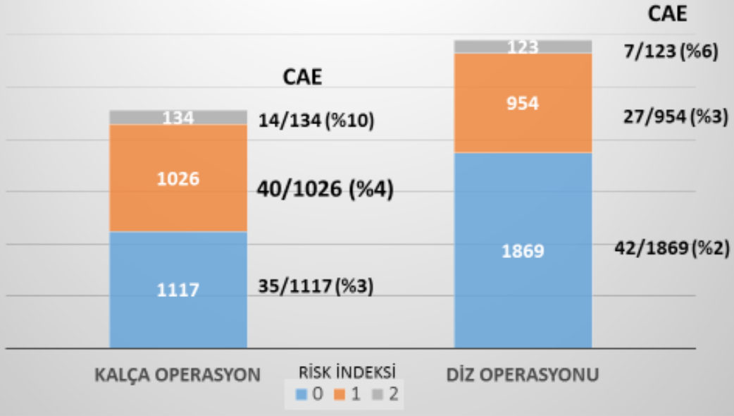
Şekil 1. Risk indekslerine göre kalça/diz operasyon sayıları ve enfeksiyon oranları
