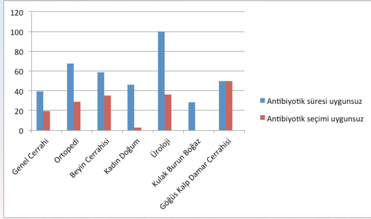
Figür 1: Branşlara göre cerrahi profilakside antibiyotik uygunsuzlukları.
