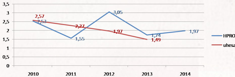
Grafik 1: Yıllara göre HPRO ameliyat kategorisinde hastanemiz ve UHESA Türkiye CAE Hızları
