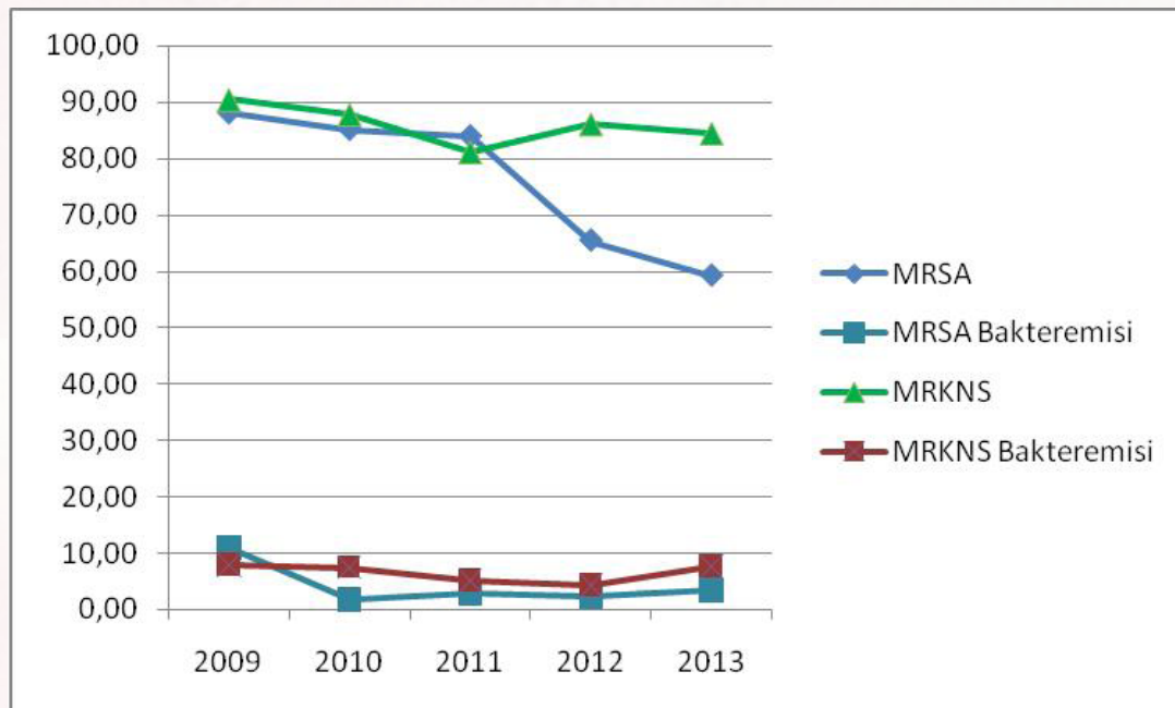
Şekil 1: MRSA, KNS oranları ve bakteriyemi oranları
